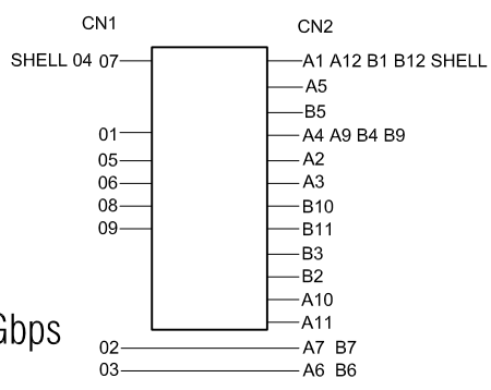
USB-C母 to USB-A公線位圖
